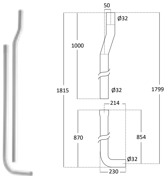
Tubo per cassetta alta esterno per vaso
