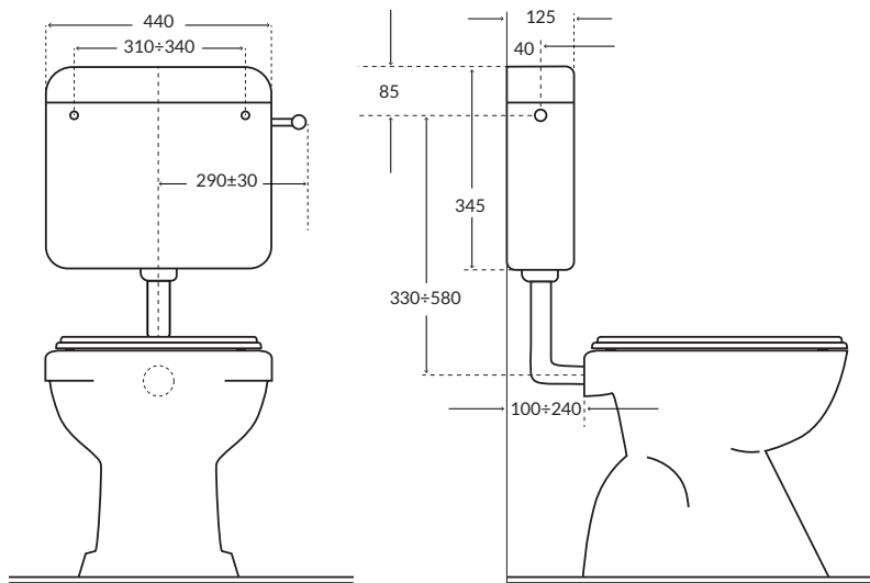
DOPPIO SCARICO DOUBLE FLUSH
