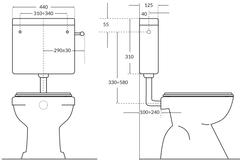
ALTA CON TUBO IN 5 PEZZI HIGH LEVEL, 5 PCS. PIPE
